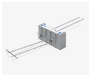
Schöck Isokorb® RT Typ Q-P positive Querkraft
