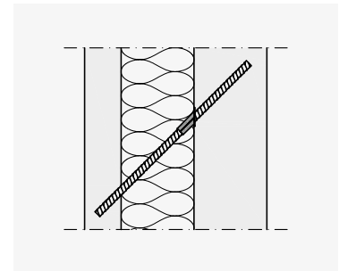
Einbau Schöck Isolink® Typ C-SD
