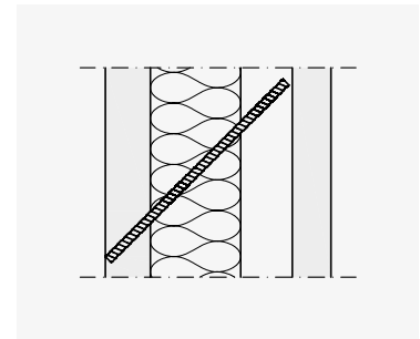
Einbau Schöck Isolink® Typ C-ED
