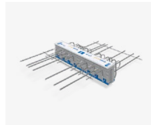
Schöck Isokorb® XT Typ K-BH
