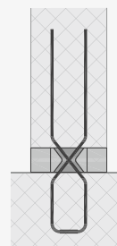
Einbau Schöck Sconnex® Typ W-N-VH
